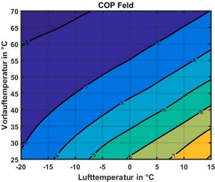
Abb. 30: EU08L bei 6kW Heizleistung
