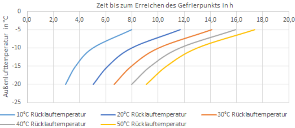
Abbildung 24: Zeitdauer bis zum Erreichen des Gefrierpunkts in den wasserführenden Bauteilen der Wärmepumpe
