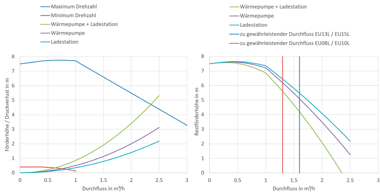
Abb. 44: Pumpenkennlinie, Anlagenkennlinie und Restförderhöhe EU08L, EU10L, EU13L, EU15L
