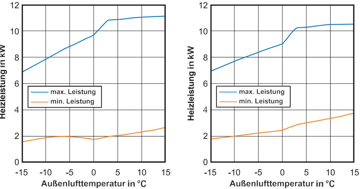
Abb. 29: EU08L bei 5K Spreizung (links: 35°C Vorlauftemperatur / rechts: 55°C Vorlauftemperatur)
