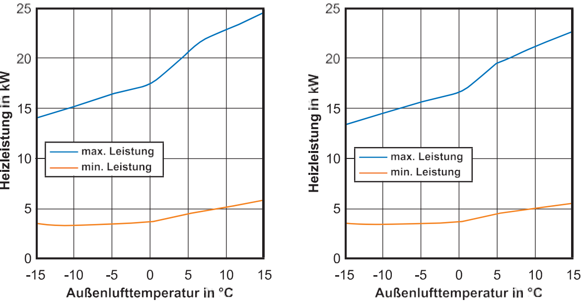
Abb. 38: EU15L bei 5K Spreizung (links: 35°C Vorlauftemperatur / rechts: 55°C Vorlauftemperatur)
