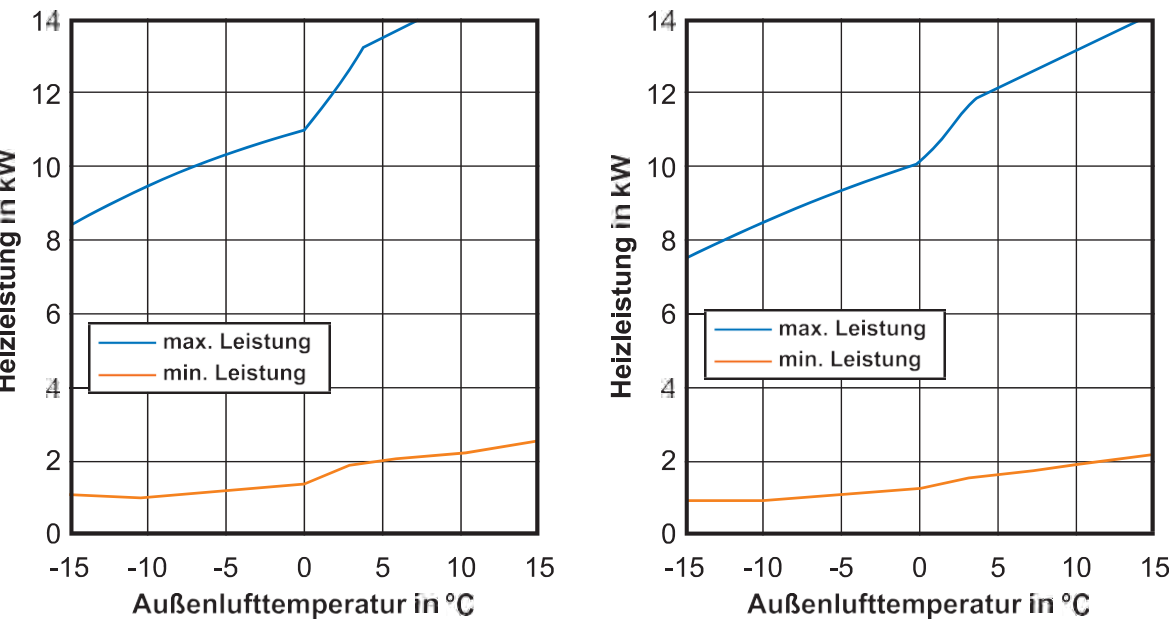
Abb. 32: EU10L bei 5K Spreizung (links: 35°C Vorlauftemperatur / rechts: 55°C Vorlauftemperatur)
