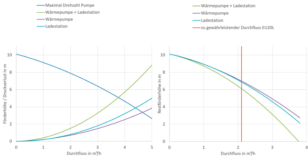
Abb. 45: Pumpenkennlinie, Anlagenkennlinie und Restförderhöhe EU20L
