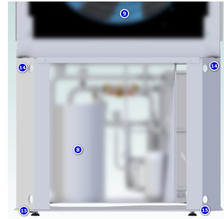
Abbildung 7: Ausstattung des Außengeräts: Ansicht hinten Kältekreis
