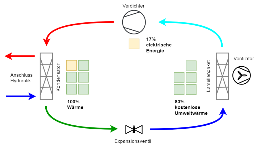
Abbildung 2: Funktionsprinzip
