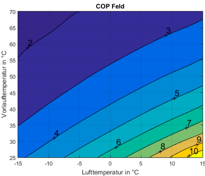
Abb. 33: EU10L bei 6kW Heizleistung
