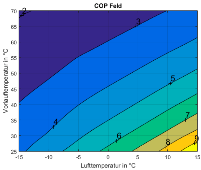
Abb. 42: EU20L bei 14kW Heizleistung
