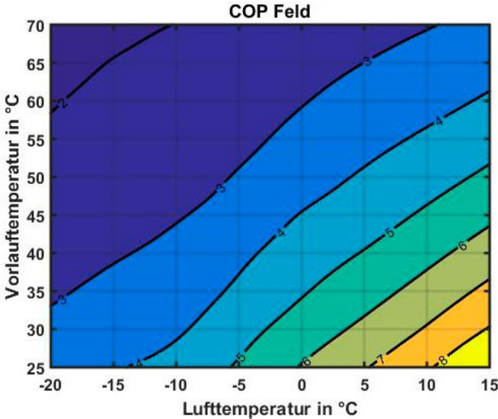
Abb. 36: EU13L bei 9kW Heizleistung
