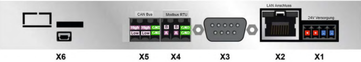
Abbildung 20: Anschlussklemmen Regelzentrale Display
