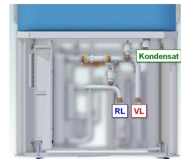
Abbildung 15: Hydraulik anschließen
