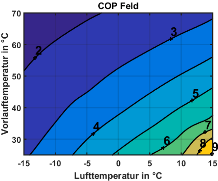
Abb. 39: EU15L bei 11kW Heizleistung
