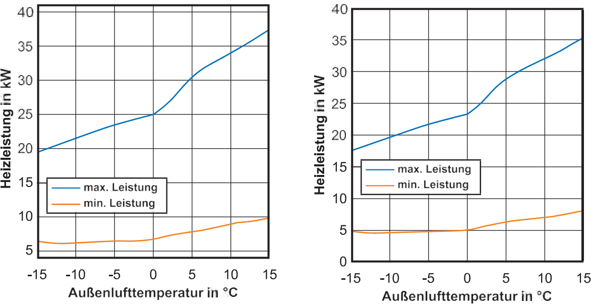
Abb. 41: EU20L bei 5K Spreizung (links: 35°C Vorlauftemperatur / rechts: 55°C Vorlauftemperatur)
