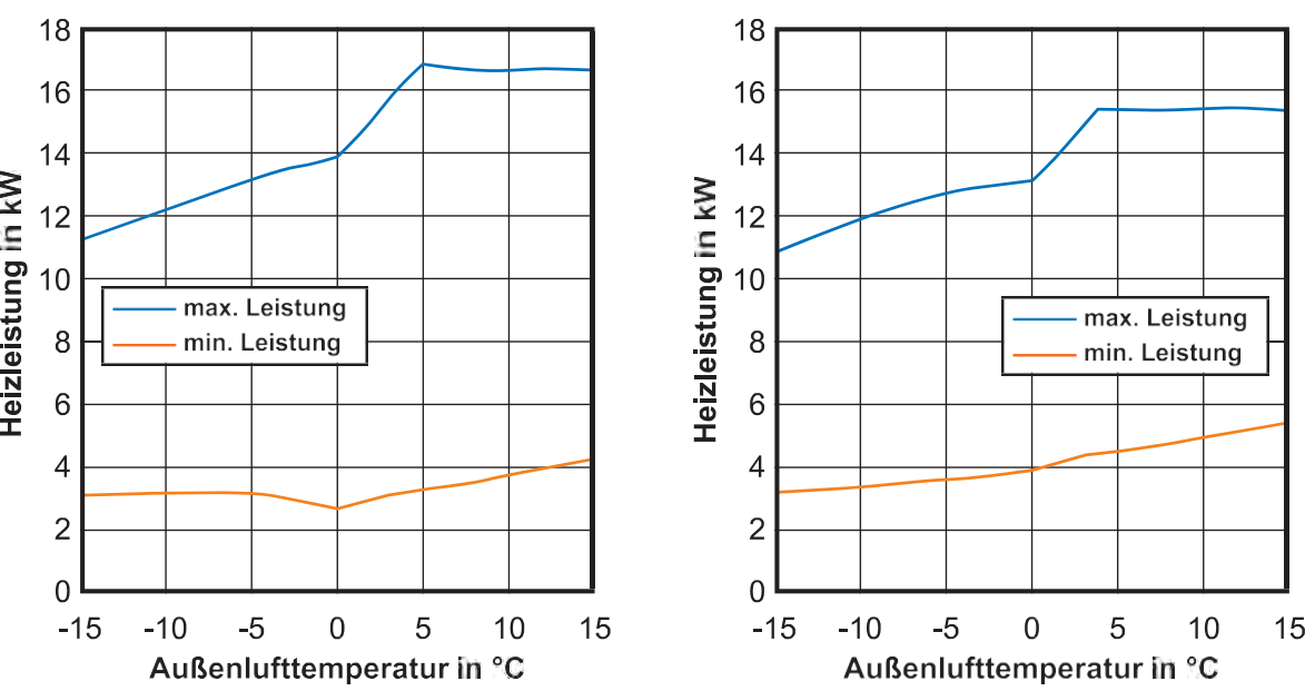
Abb. 35: EU13L bei 5K Spreizung (links: 35°C Vorlauftemperatur / rechts: 55°C Vorlauftemperatur)
